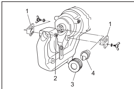
► 1. Dévissant 2. Écrou et boulon de fixation 3. Écrou de retenue du poinçon 4. Poinçon rond
